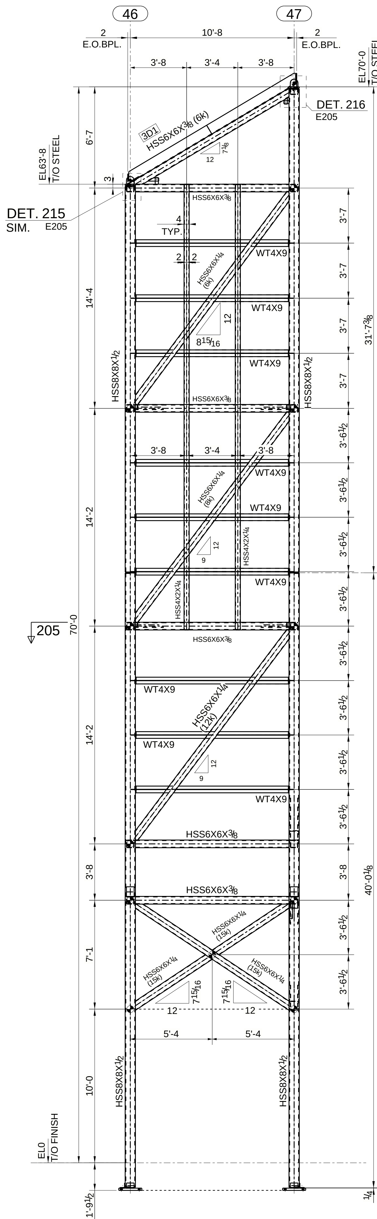
SECTION 201 - 201
