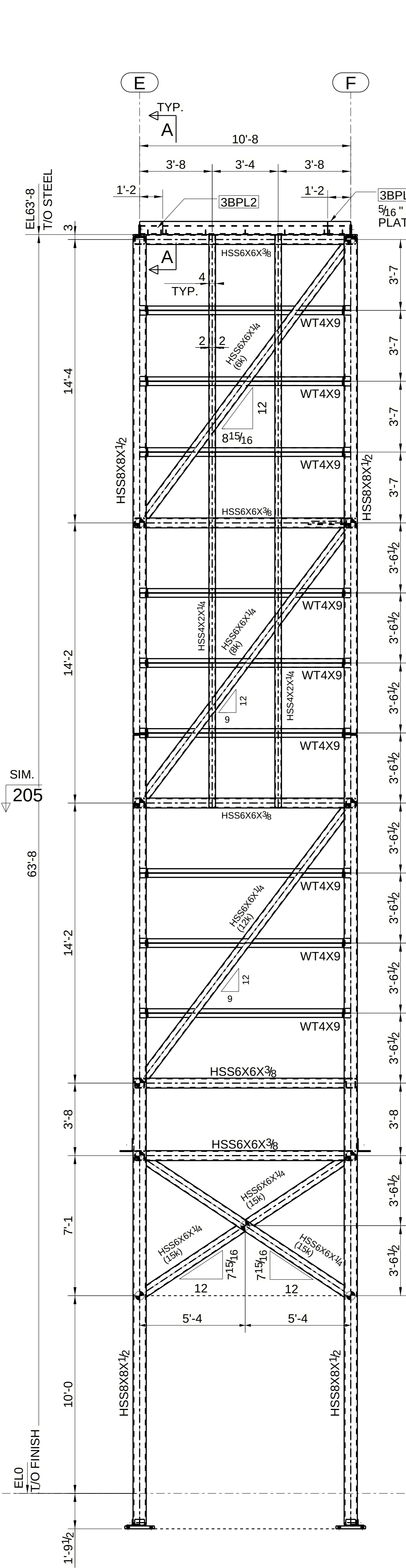
SECTION 202 - 202
