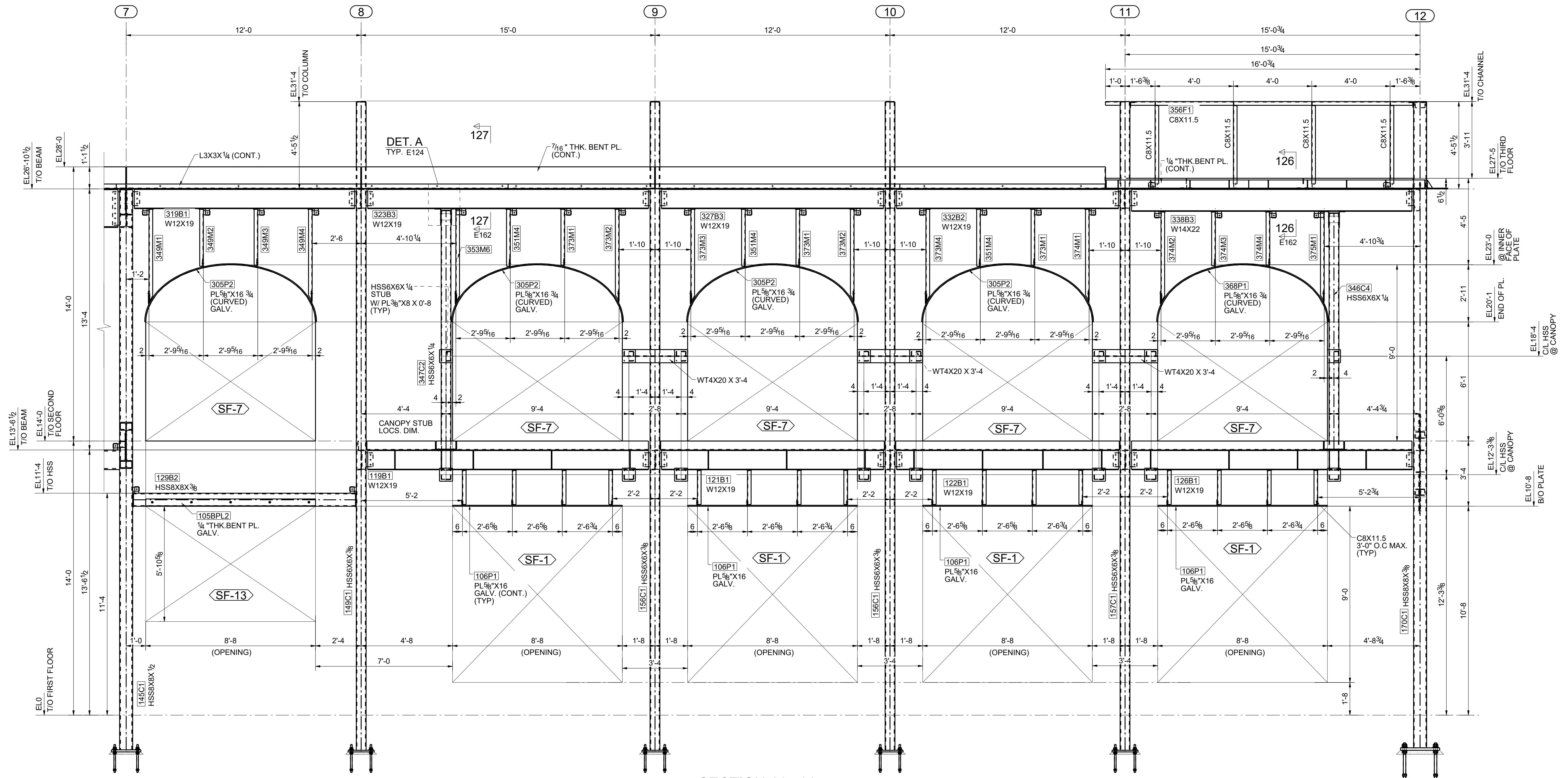
SECTION 11 - 11 E101 (REFER : EAST ELEVATION S-301)
