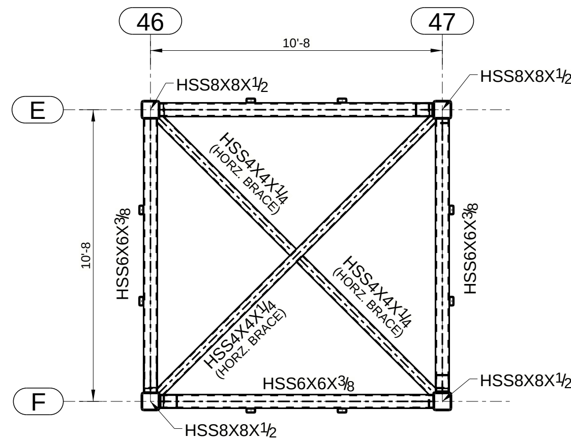
SECTION 205 - 205
